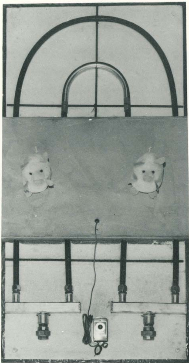
※豚舎床面暖房施工カット・モデル
